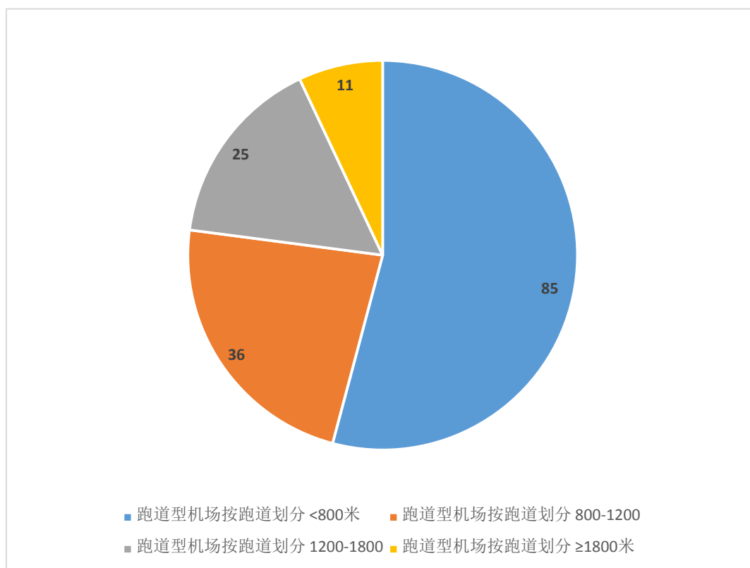
图 7 全国颁证跑道型通用机场按照跑道划分对比图
