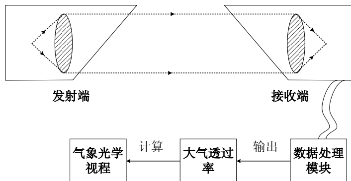
图 1 大气透射仪通用组成结构示意图
